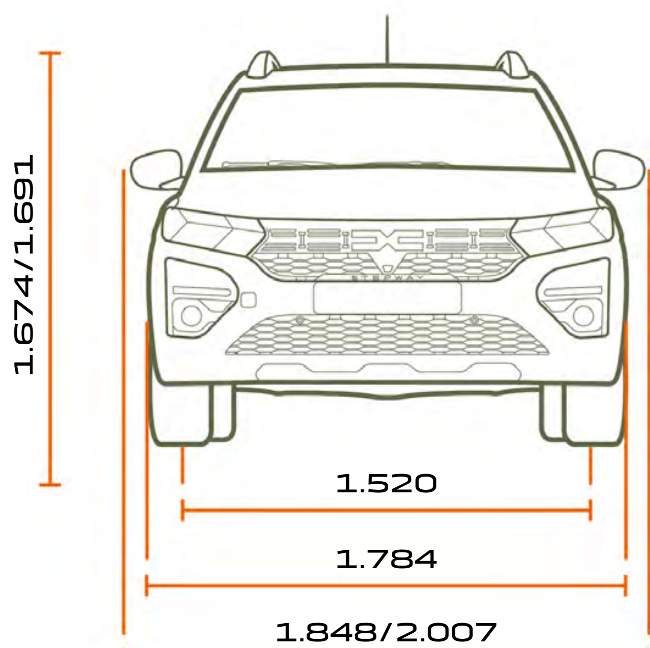
FRONTANSICHT 5- UND 7-SITZER
