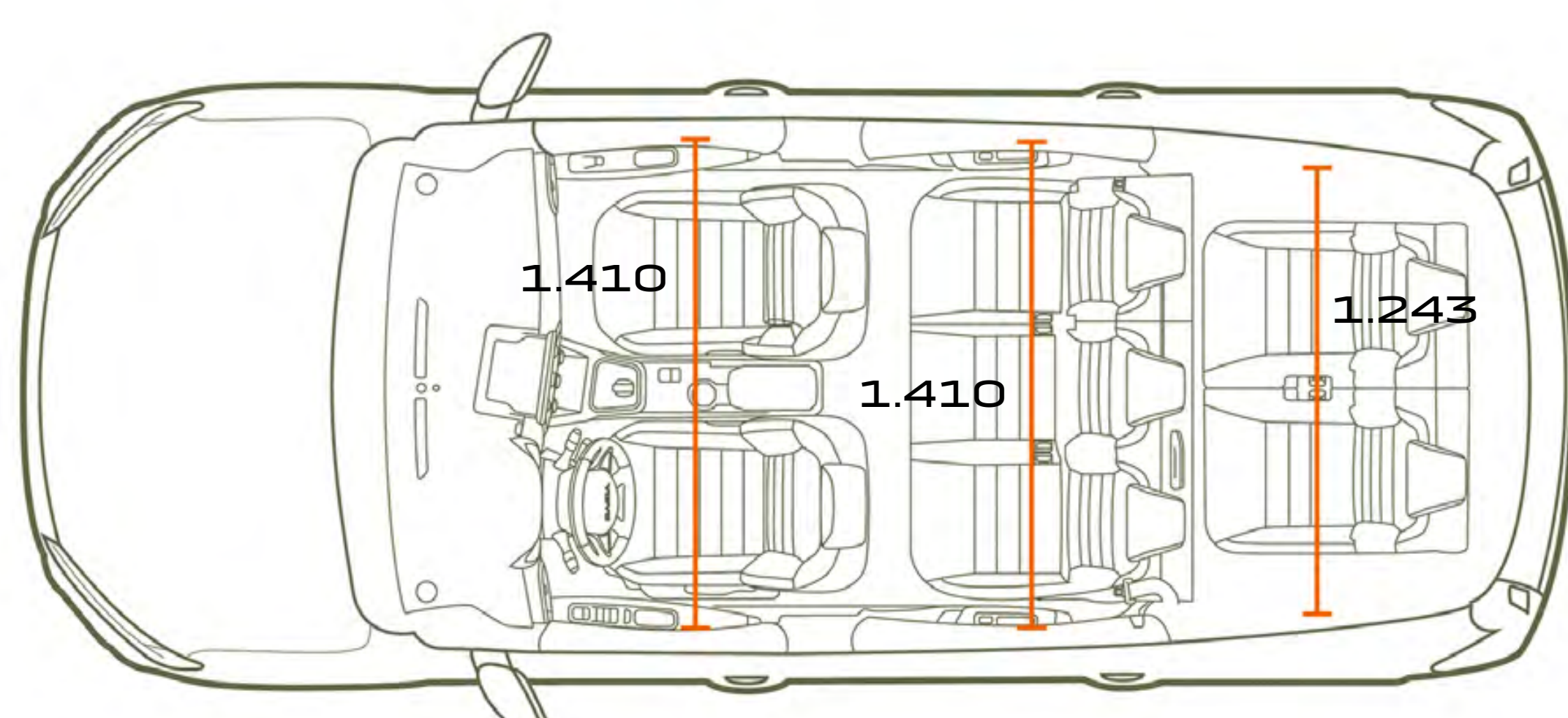
ANSICHT VON OBEN 7-SITZER
