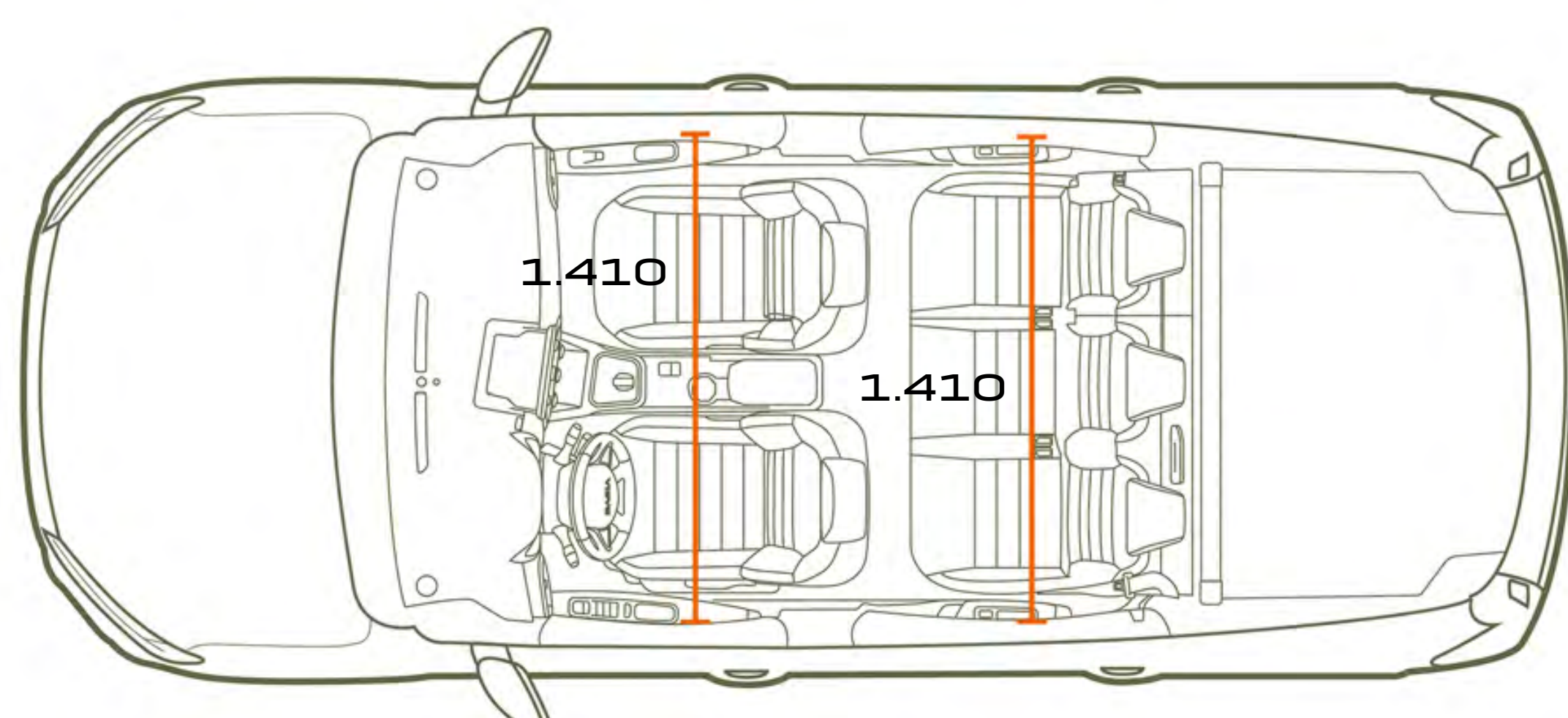
ANSICHT VON OBEN 5-SITZER
