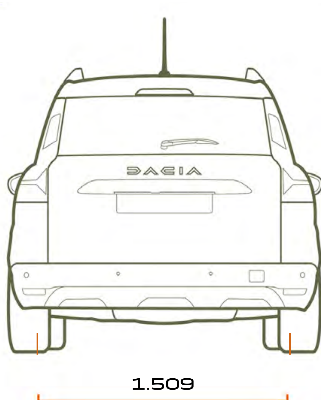
HECKANSICHT 5- UND 7-SITZER
